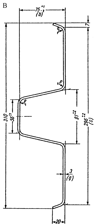
Załącznik 11.4. Profilowana taśma stalowa typu B, wg L. Mikołajków: Drogowe bariery ochronne, WKiŁ, 1983
