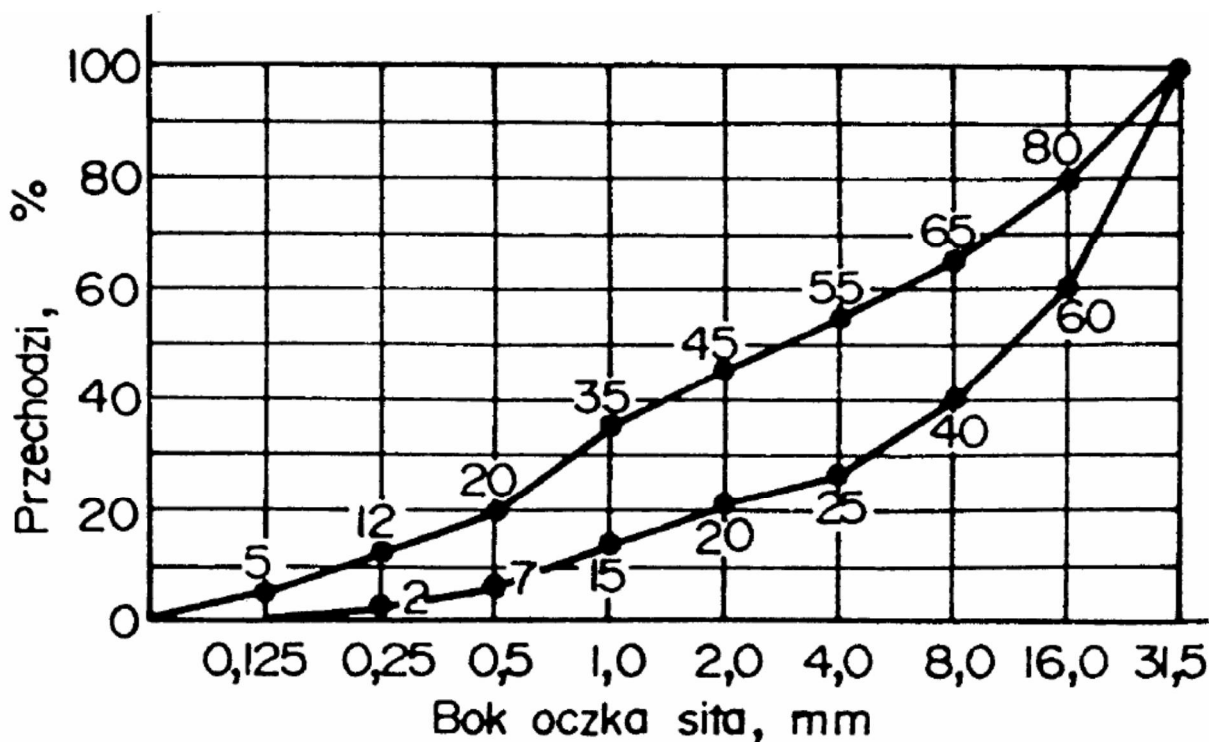
Rysunek 1. Graniczne krzywe uziemia do chudego betonu od 0 do 31,5 mm.
