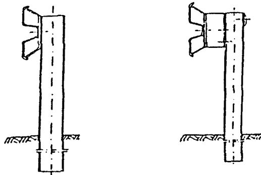
Załącznik 11.3. Zasady określania wysokości prowadnicy bariery nad poziomem terenu,
